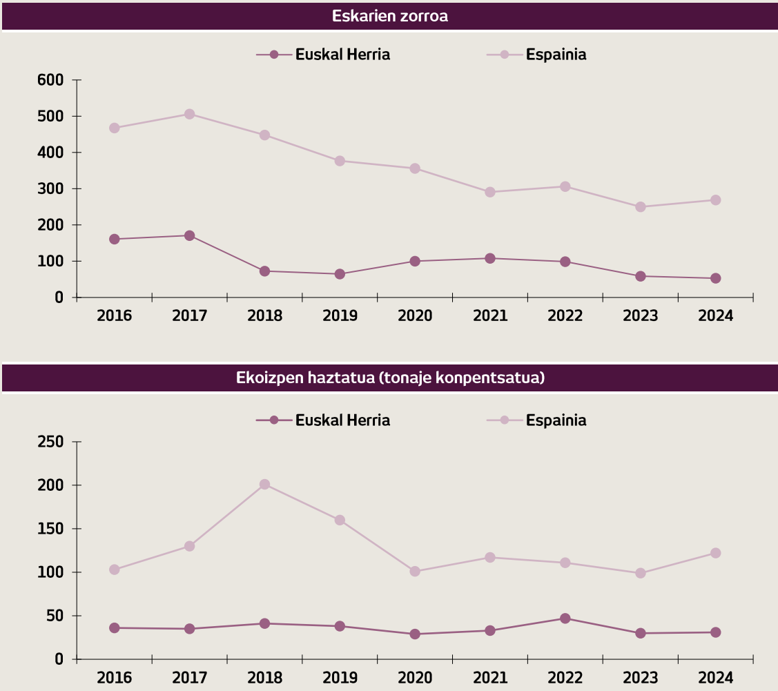
15. grafikoa Ontzigintzako eskaera-zorroaren eta ekoizpen haztatuaren bilakaera (mCGT)
